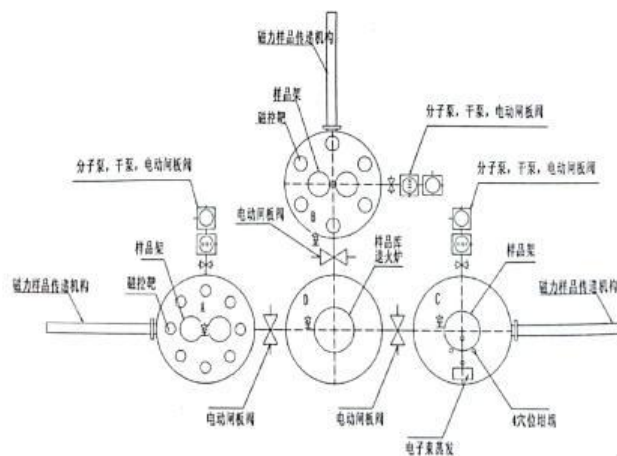
工作原理图
