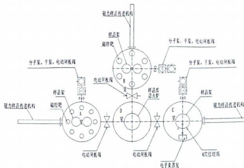
工作原理图
